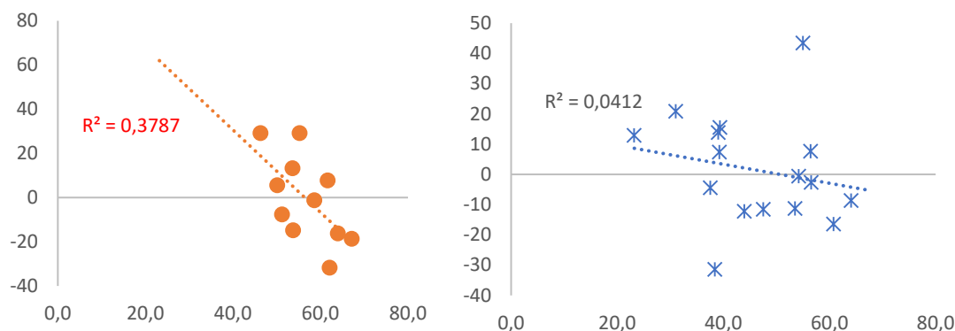
Figur 7. Relationen mellan externfinansieringsgrad (%; horisontell axel) och den relativa avvikelsern (%) från den linjära relationen mellan total finansiering och bibliometriskt index (vertikal axel). Vänster figur avser äldre universitet och den högra nya universitet och högskolor.
